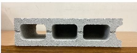
[端部のみ貫通]
