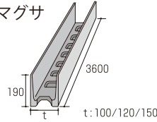
GRCマグサ
